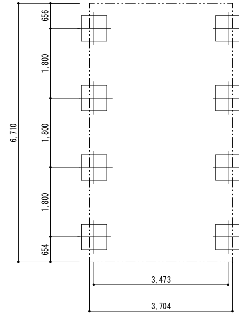
■ 基礎配置図
