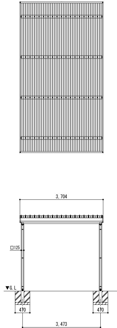
■ 立面図
